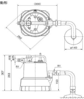
■外形寸法図 単位: mm 非自動形
